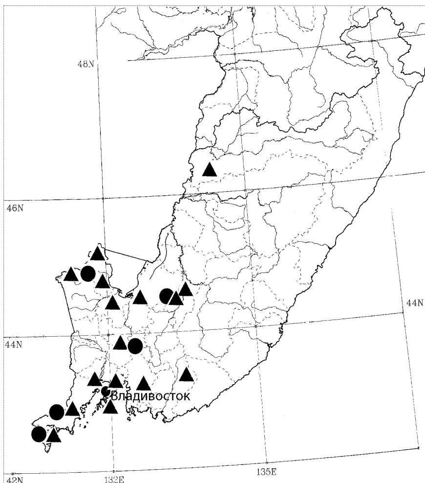
Рис. 1. Карта распространения в Приморском крае H. diomphalia : ● – по литературным данным (Калинина, 1977), ▲ – изученный материал
